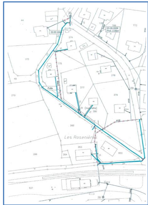
Canalisations eau propre :
